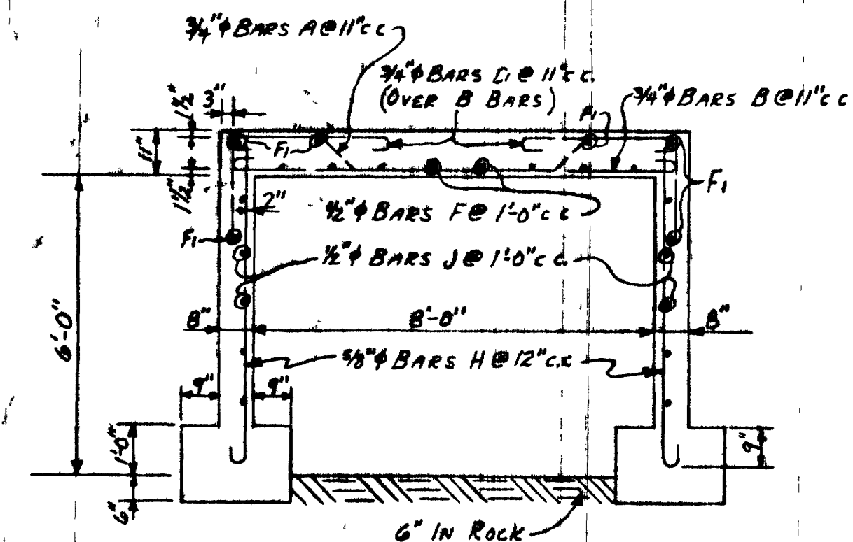
FILL SECTION 11'-15'
